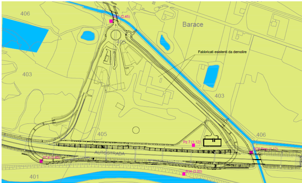
Figura 33 – Ubicazione piezometri
