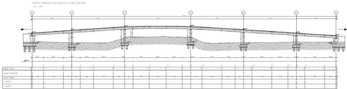
Sovrappasso di uscita- profilo longitudinale
