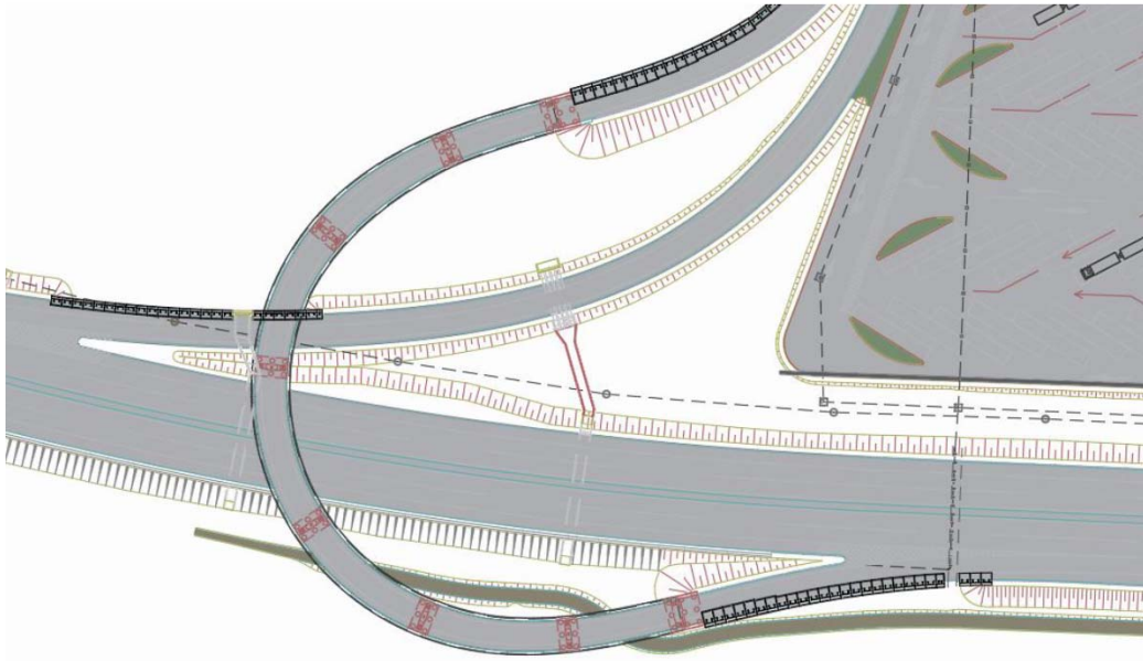
Sovrappasso di ingresso-planimetria
