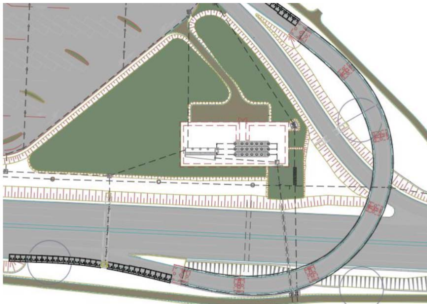
Sovrappasso di uscita-planimetria
