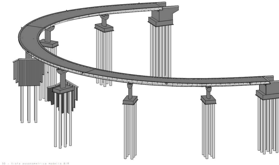
Vista assonometrica Rampa di Ingresso
