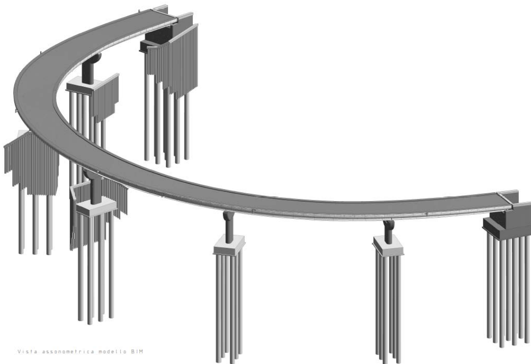
Vista assometrica Rampa di uscita
